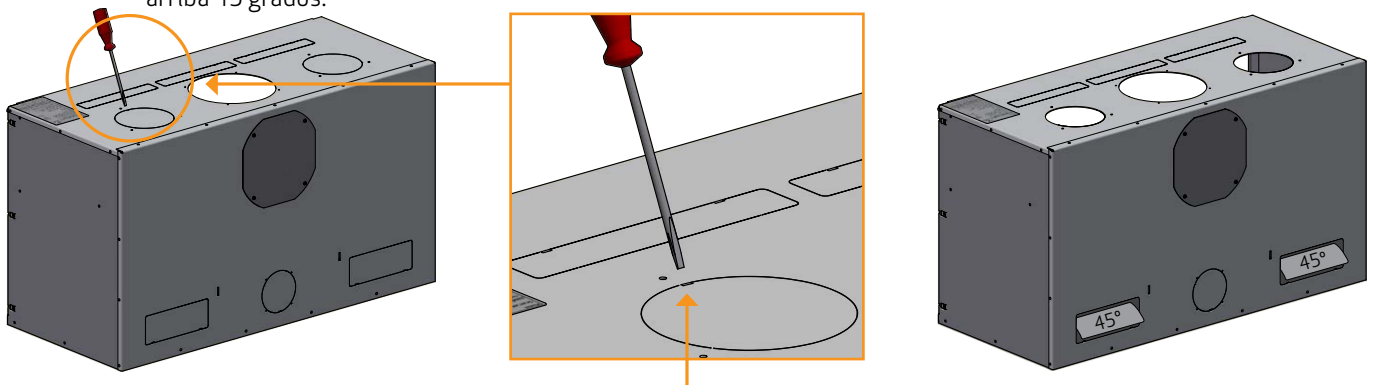
Cassette sin placas de cubierta para el conexión de convección
